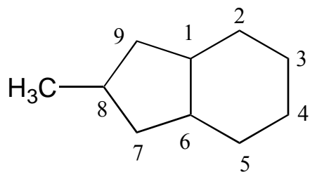
8-metilbiciklo[4.3.0]nonán
